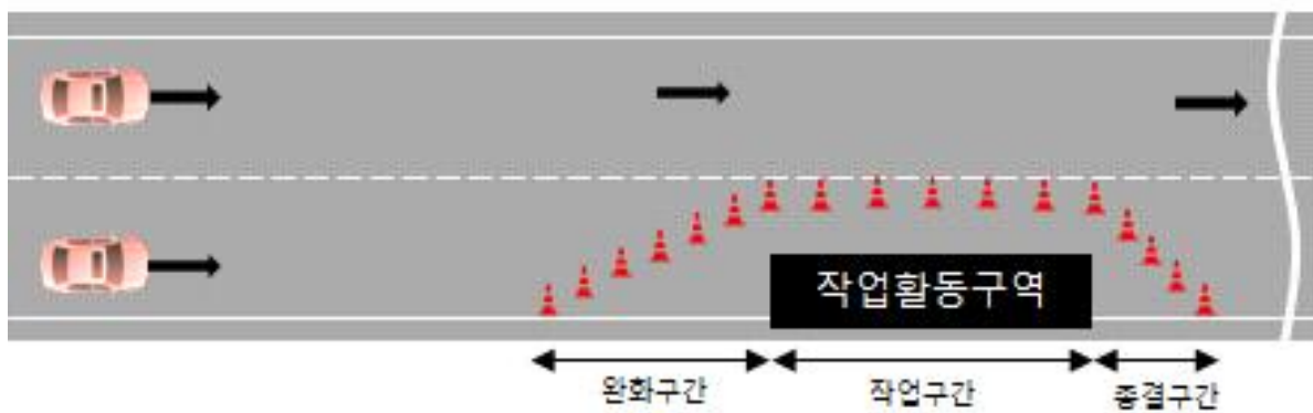
<그림 2.1> 차로 완전 차단
