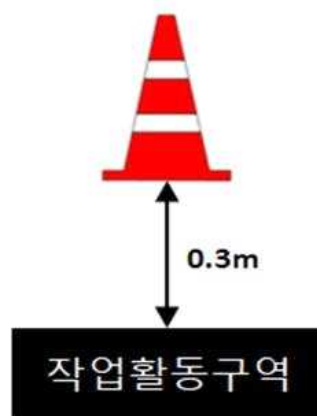
<그림 3.4> 측방향 완충구간
